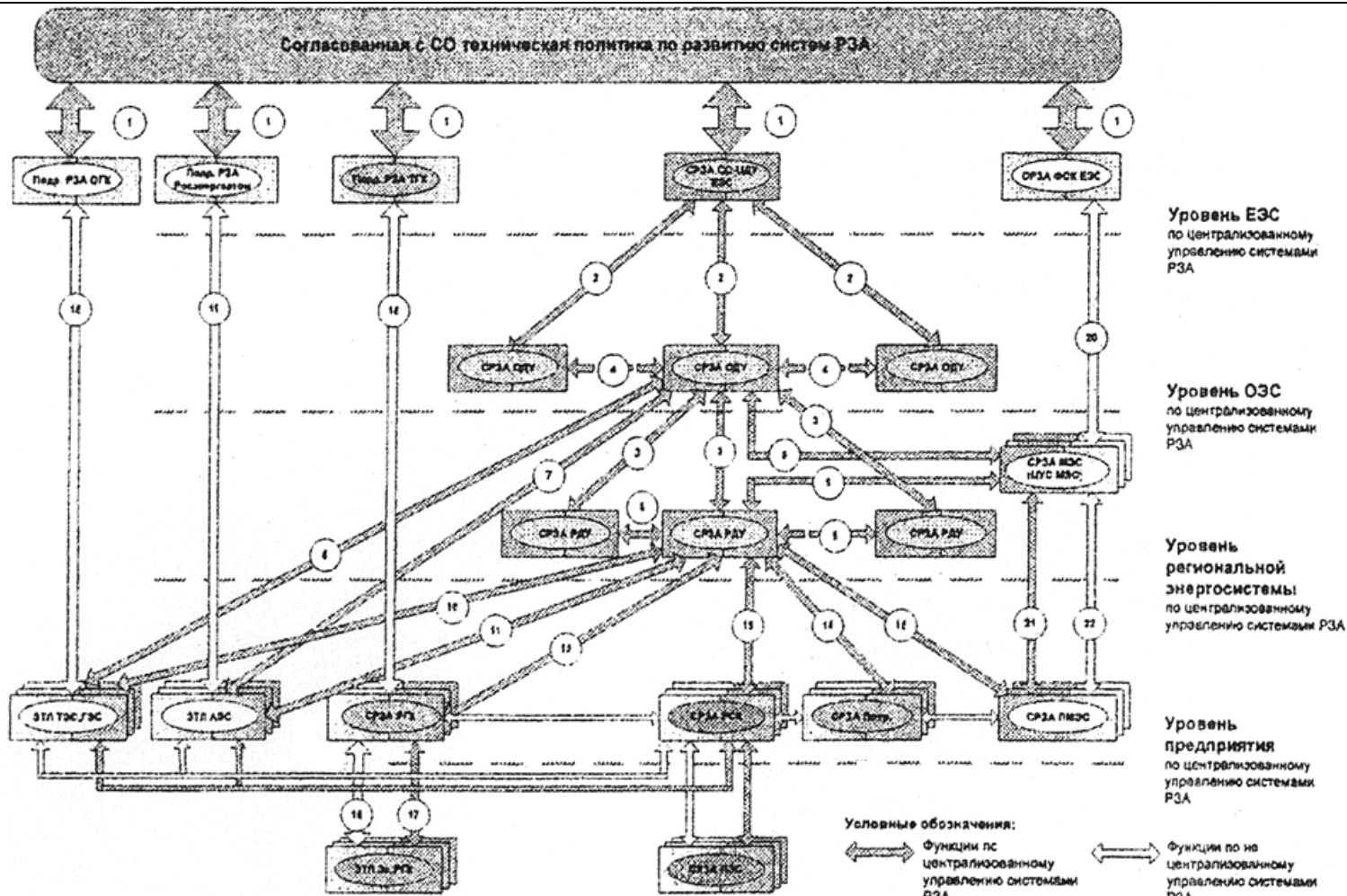
Рис.1 Принятая в Стандарте структурная схема взаимодействия служб РЗА
