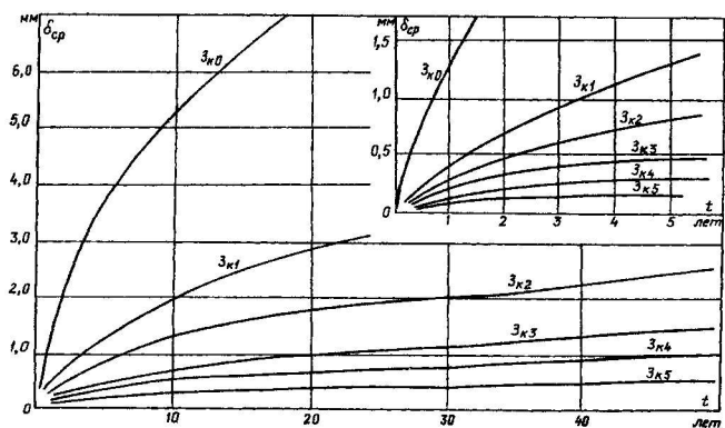
Рис. П3.2. Рост средней глубины грунтовой коррозии стали
