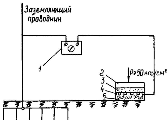
Рис. 9. Схема измерения сопротивления основания:
