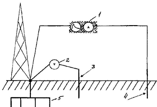
Рис. 6. Схема измерения сопротивления заземлителей опор ВЛ и молниеотводов:
